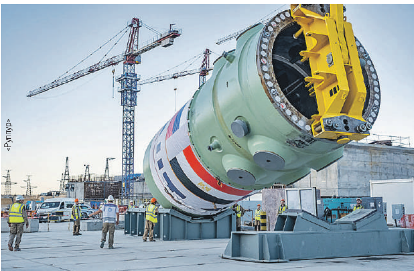
В Египте установили в проектное положение корпус реактора первого энергоблока АЭС «Эль-Дабаа».
